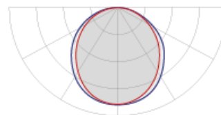
Curva fotometrica
